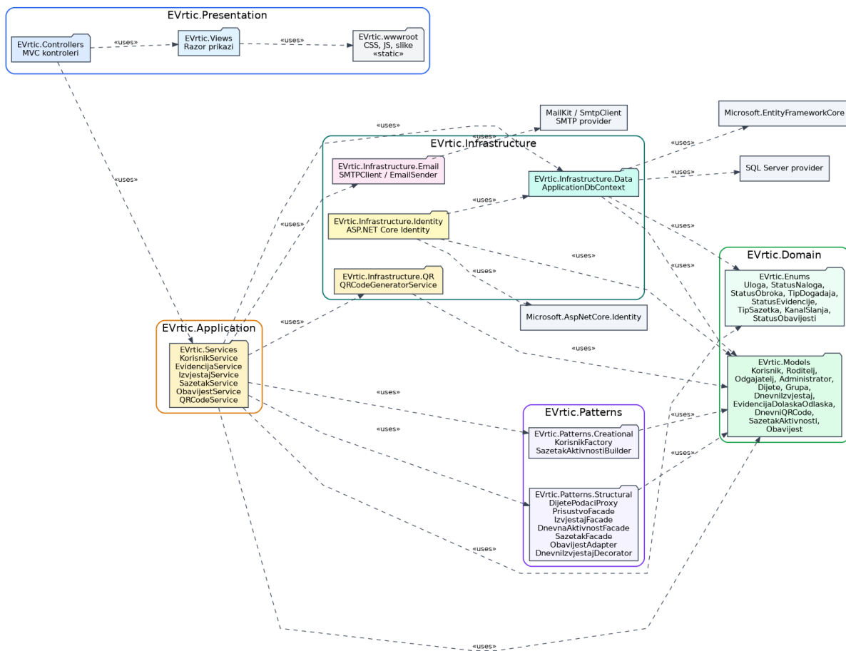
Dijagram paketa - eVrtić sistem
